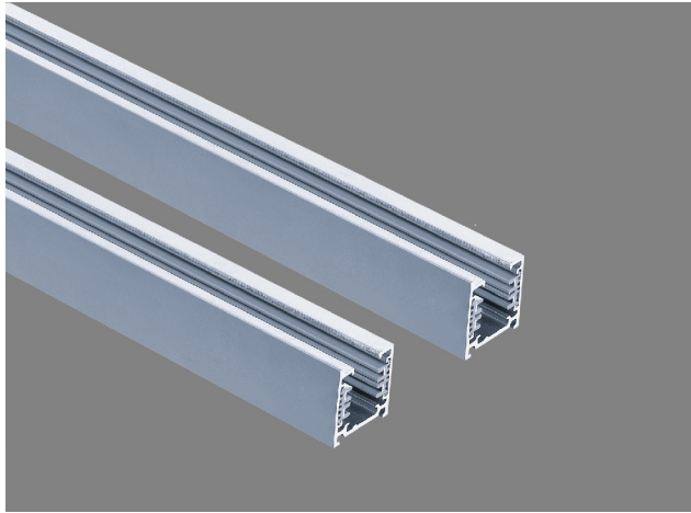
HT4-1M · 2M · 3M 3-Circuit Track(Surface Mounted) 220V · 16A
